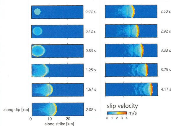
鉛直横ずれ断層における超せん断破壊(supershear rupture)の場合の破壊伝播のスナップショット(すべり速度) Snapshot of supershear rupture propagation for a lateral slip on a vertical fault plane.
