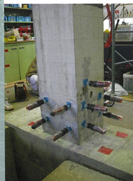
樹脂によるひび割れ補修 Epoxy Resin Injection into Cracks
