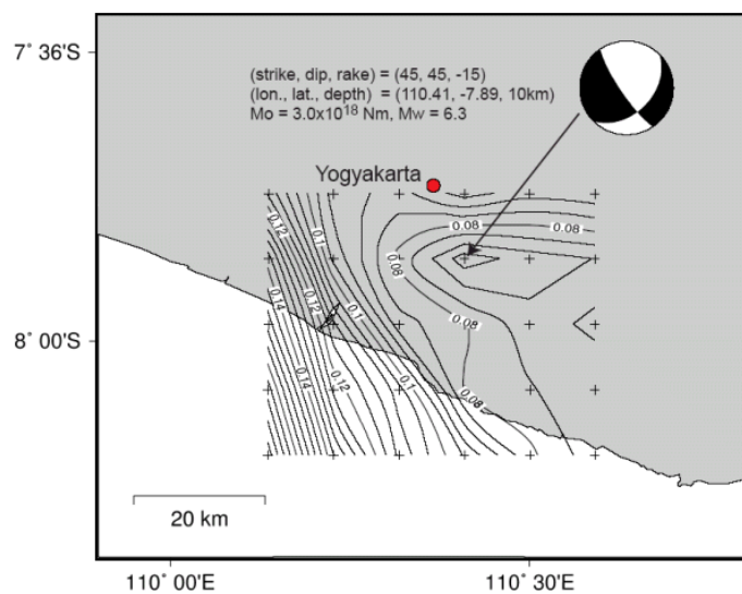
図-9 震源位置の同定（防災科学研究所国際地震観測管理室による）
