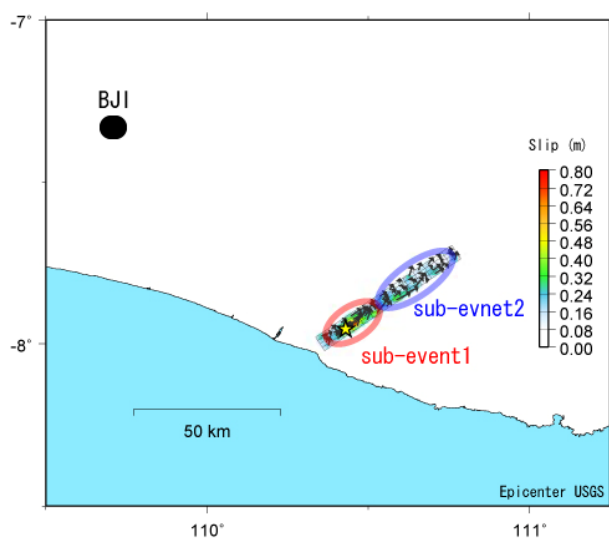
(b) 震源位置
