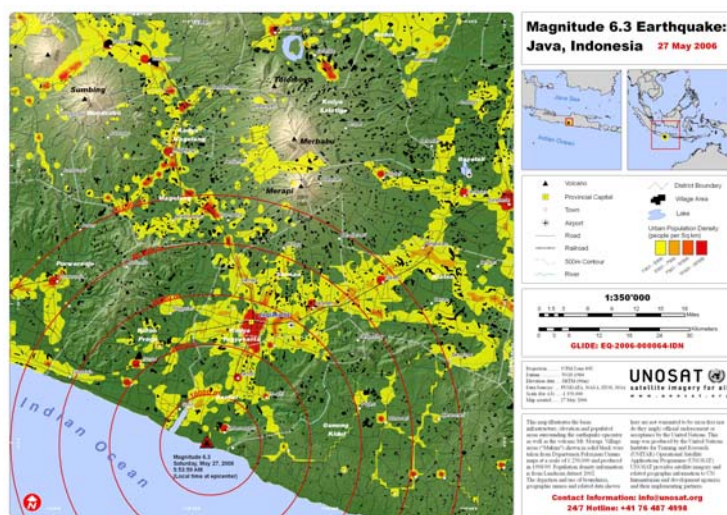
図-3 UNOSATによる震源速報
