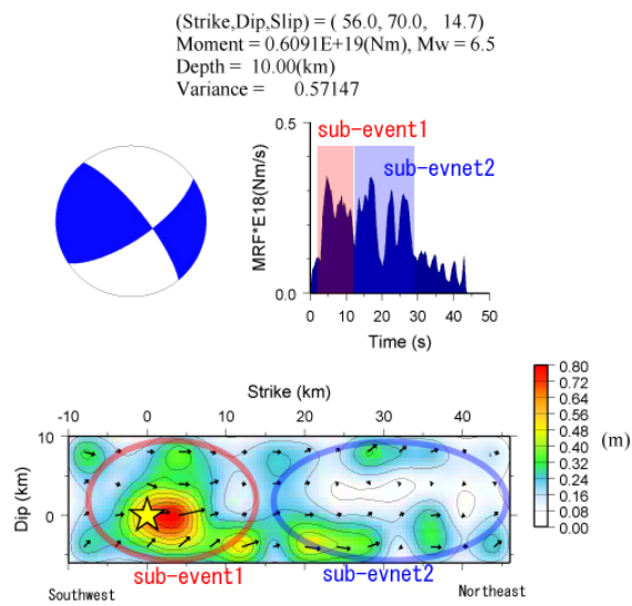
(a) 地震規模と震源
