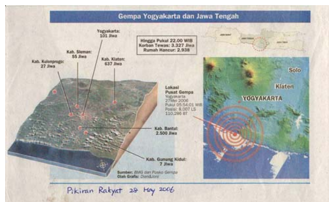
図-2 地震発生の速報 (Pikiran Rakyat, 5月28日, 2006)
