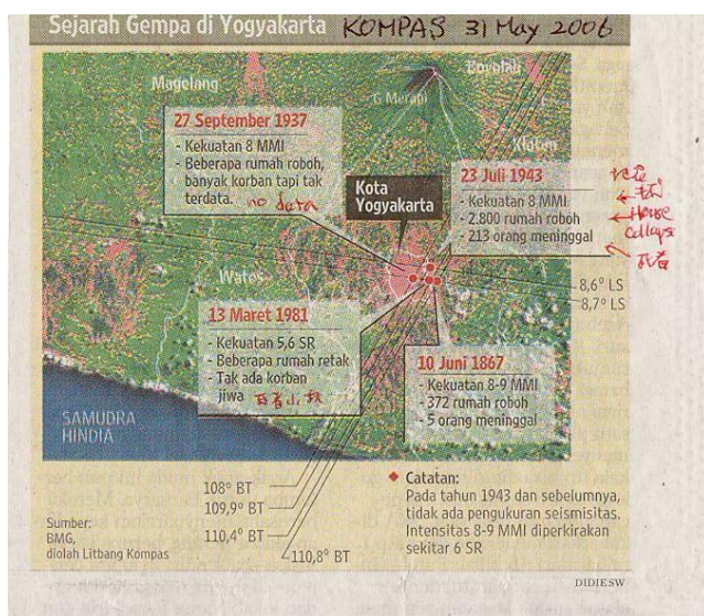
図-10 Yogyakarta 近郊での過去の大型地震（KOMPAS, 5月31日, 2006）
