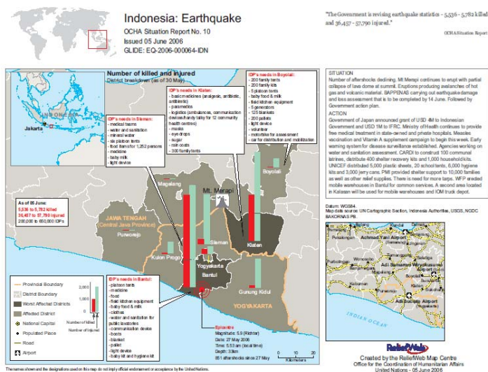
図-5 OCHAによる死傷者・負傷者の数
