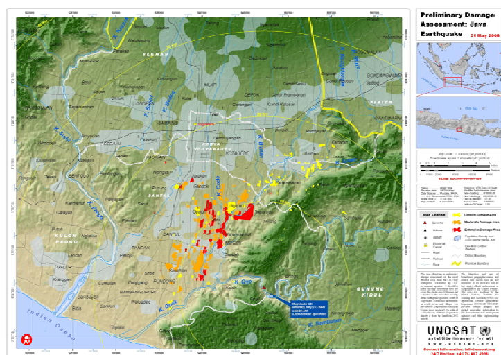
図-4 UNOSATによる震源と被災情報
